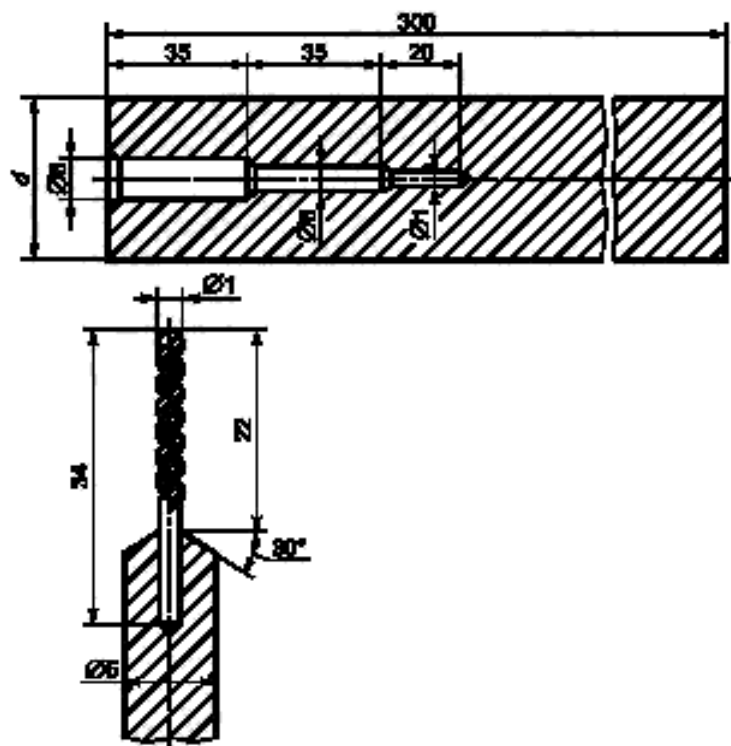
Рисунок Б.1 — Стандартный образец для настройки чувствительности аппаратуры
