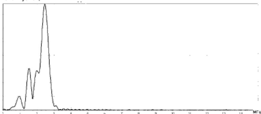
Рисунок 1 – Амплитудный спектр для резьбы СОП.
