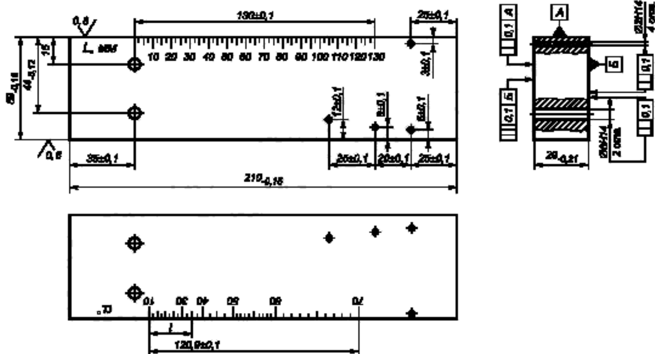
Рисунок 3 — Стандартный образец СО-2Р
