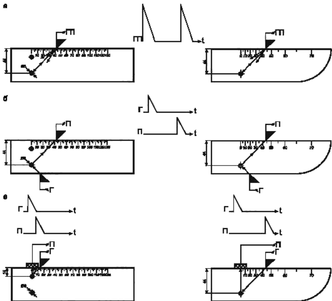
Г — вывод к генератору дефектоскопа; П — вывод к приемнику дефектоскопа
