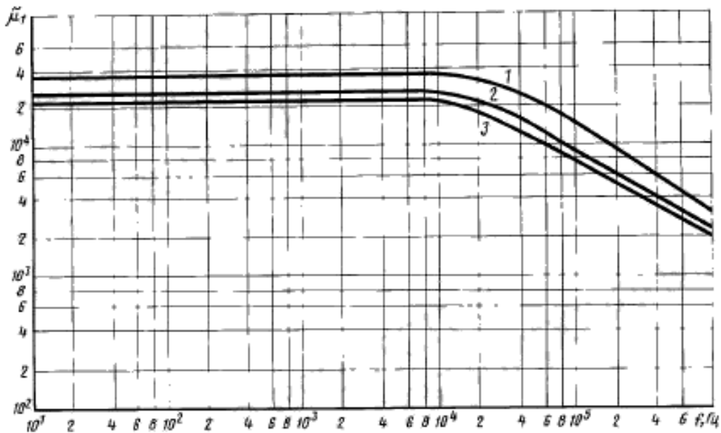
Зависимость \tilde{\mu} от частоты для сплавов и лент толщиной 0,02 мм марок: 1 — 83НФ; 2 — 80НХС; 3 — 79НМ
