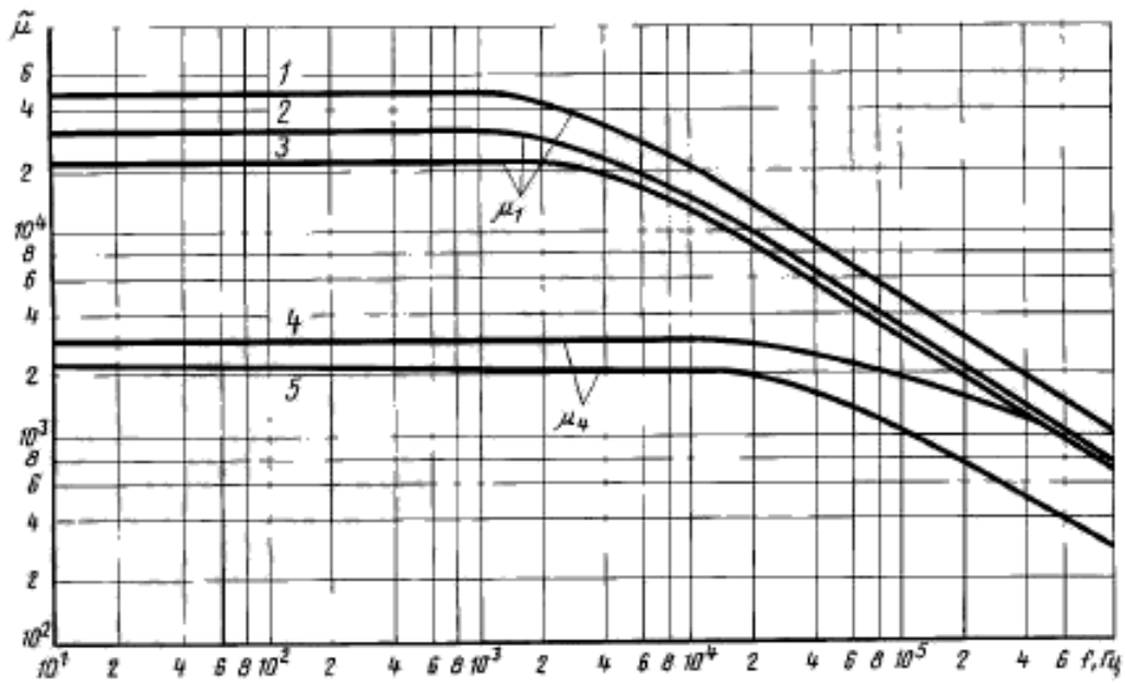
Зависимость \tilde{\mu} от частоты для сплавов и лент толщиной 0,05 мм марок: 1 — 81НМА и 83НФ; 2 — 80НХС; 3 — 79НМ; 4 — 50НХС; 5 — 50Н
